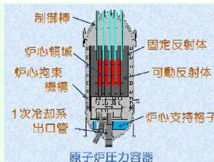
図1b HTTRの原子炉圧力容器 HTTRの画像検索結果より転載
