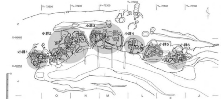
図5 製鉄炉分布全体図 (1/400)
